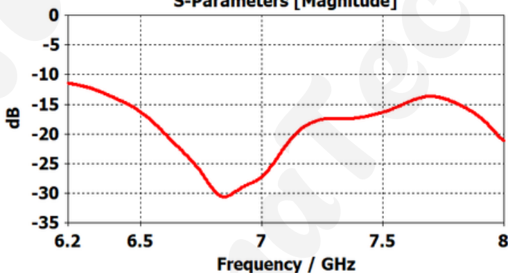
S-Parameters [Magnitude]
